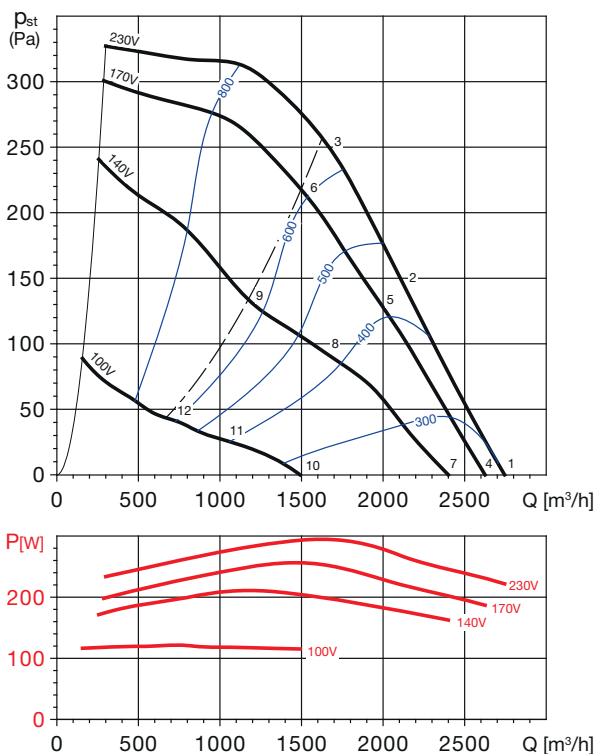
CTHB/4-250 N
