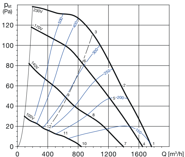
CTHB/6-250 N
