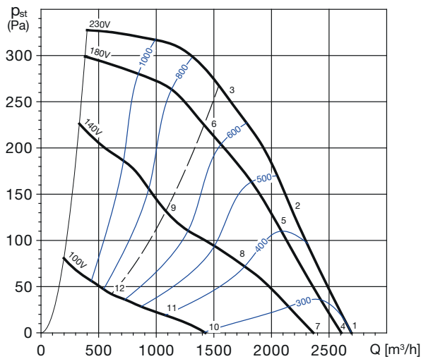
CTVB/4-250 N
