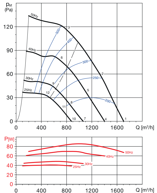
CTVT/6-250 N
