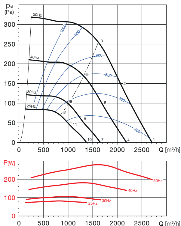
CTHT/4-250 N
