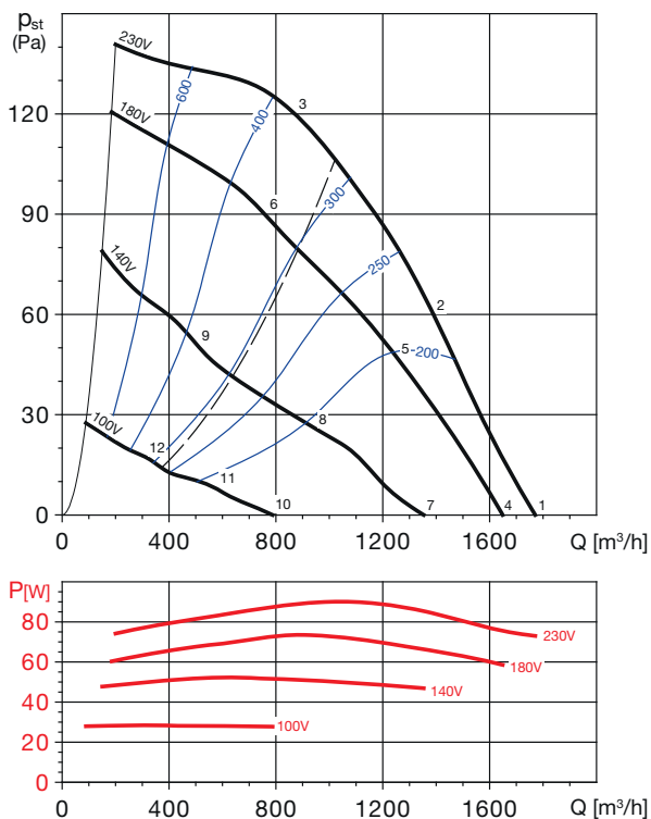
CTVB/6-250 N
