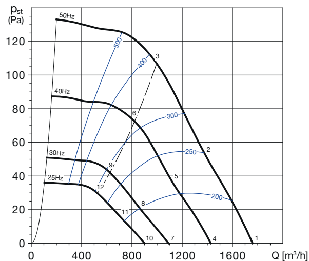
CTHT/6-250 N
