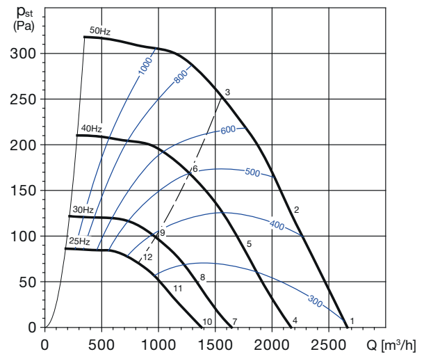
CTVT/4-250 N
