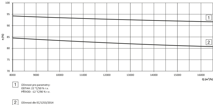
DUOVENT® MODULAR DV 14500 – účinnost rekuperace
