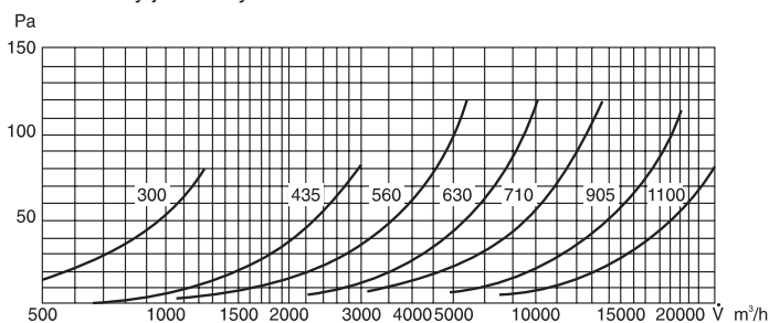
Tlakové ztráty jednotlivých velikostí tlumiče
